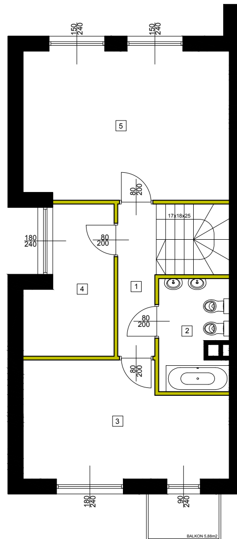
PIĘTRO
